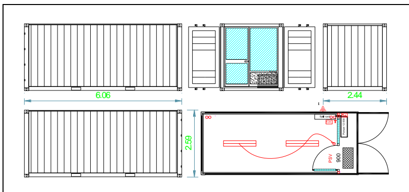
Container Maritime 20' Aménagé "Sécurisé"
