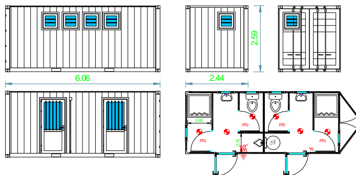
Container Maritime 20' Aménagé "Sanitaire H/F"
