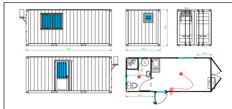
Container Maritime 20' Aménagé "Standard + Salle de Bain"
